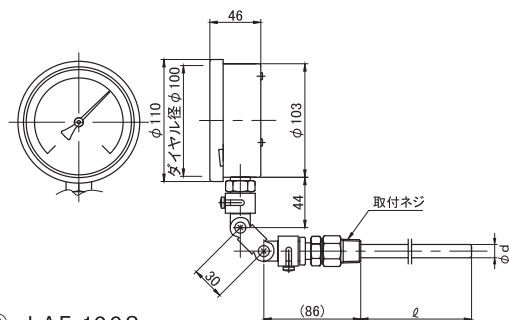
図面 ⑨ LAF-100S
